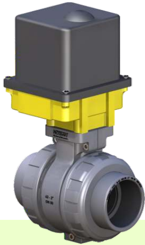
U-P.V.C. Küresel Su Vanası U-P.V.C. Water Ball Valve Dişli / Female Thread Basınç / Pressure : PN 10 Küre Contası / Seals : HDPE O-Ringler / O-Rings : EPDM
